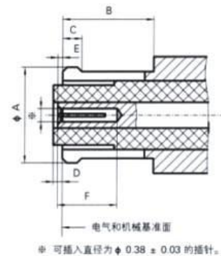
SMP系列插孔 接触件连接器界面
