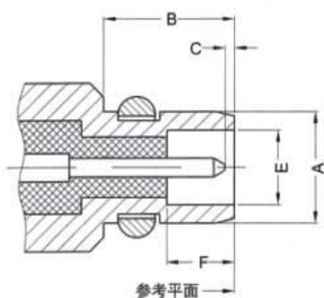
插头(Plug)
