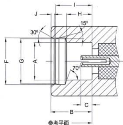
插座(Jack)
