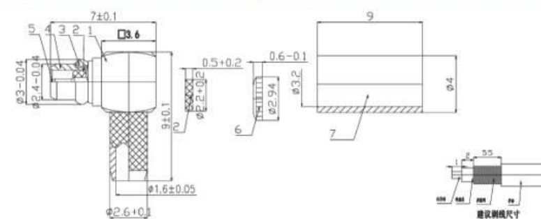
MMCX-JW1.5
