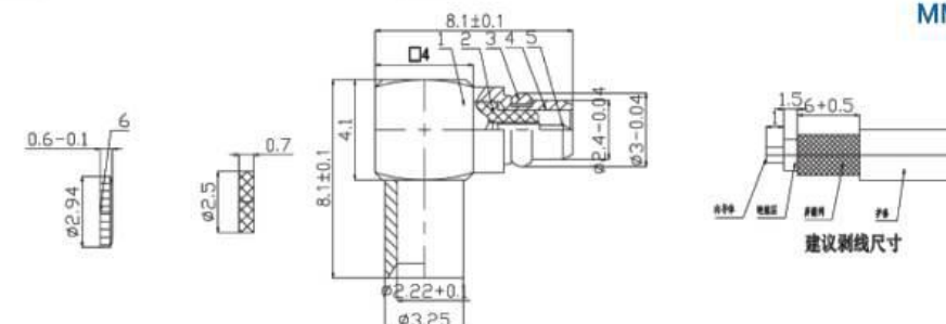
MMCX-JWB2
