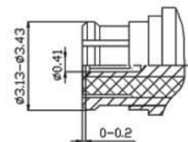
Jack(Female)
